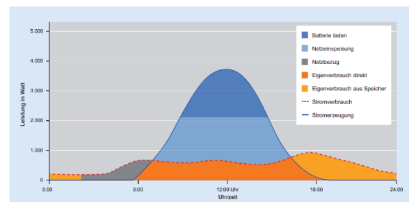
Eigenverbrauch mit Speicher (Quelle: Energieagentur NRW)
