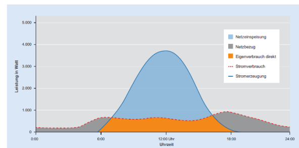
Eigenverbrauch ohne Speicher (Quelle: Energieagentur NRW)
